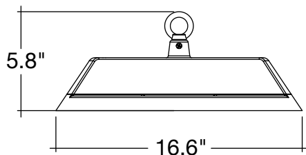
Pendant Mount
