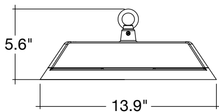
Pendant Mount
