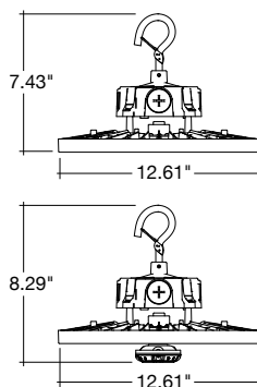
Pendant Mount
