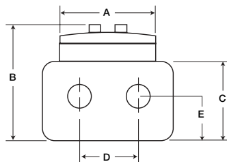
GRSS Dimensions
