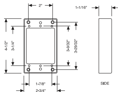
CAT. NOS. 5399-0, 5403-0
