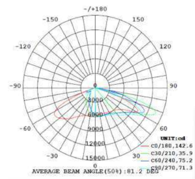
TK-SAL4-180W-T4-40K
