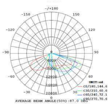
TK-SAL4-180W-50K
